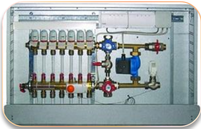
Поквартирные системы отопления
