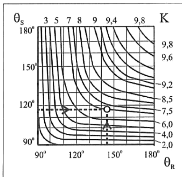
Рисунок 11.8 - Номограмма для определения расчетных значений параметра K
