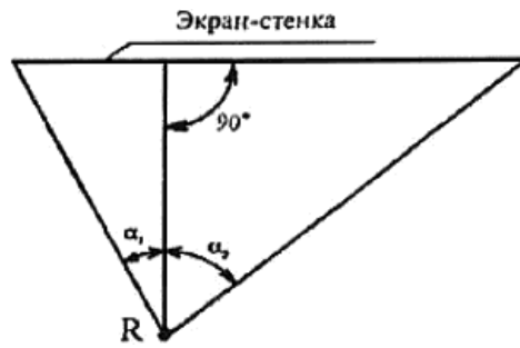
Рисунок 11.5 - Схема расчета экрана ограниченной длины
