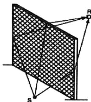
Рисунок 10.1 - Различные пути распространения звука вокруг экрана
