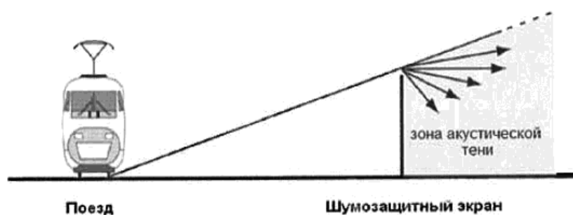
Рисунок 10.2 - Зона акустической тени за экраном
