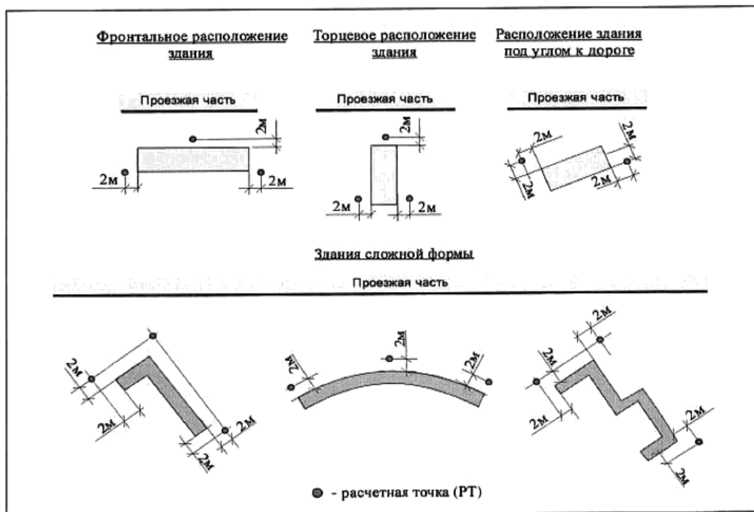
Рисунок 7.1 - Примеры расположения расчетных точек около зданий
