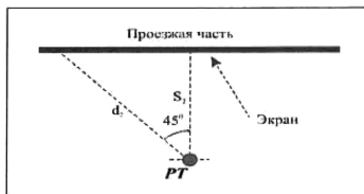
Рисунок 7.4 - Схема для определения расчетных расстояний S_2 и a_2
