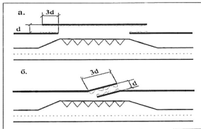
а) - контр-экран; б) - дубль-экран
