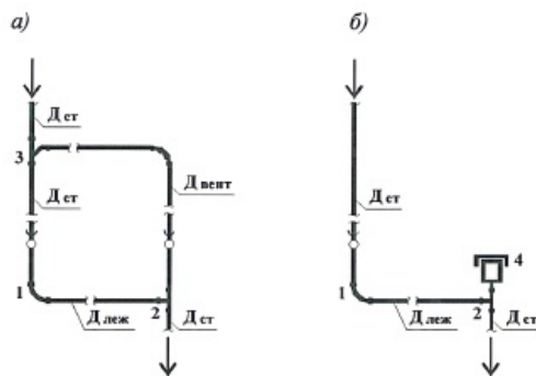
а) с устройством вентиляционного трубопровода (байпаса); б) с установкой автоматического противовакуумного клапана
