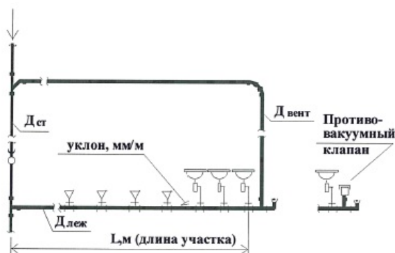
Рисунок 11.2 - Схема устройства длинной горизонтальной разводки
