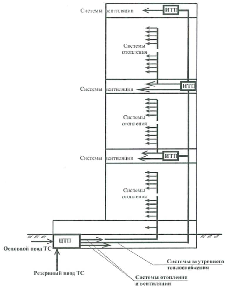
Рисунок 5.1 - Схема теплоснабжения высотного здания от централизованного источника
