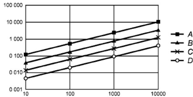
Рисунок А.3 - Классы герметичности (см. ЕН 1507 [5] и ЕН 12237)
