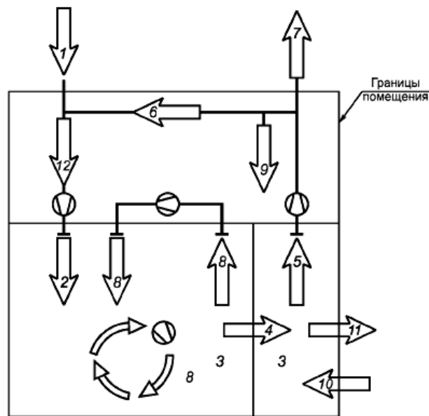
Рисунок 1 - Типы потоков воздуха. Номера позиций соответствуют таблице 2
