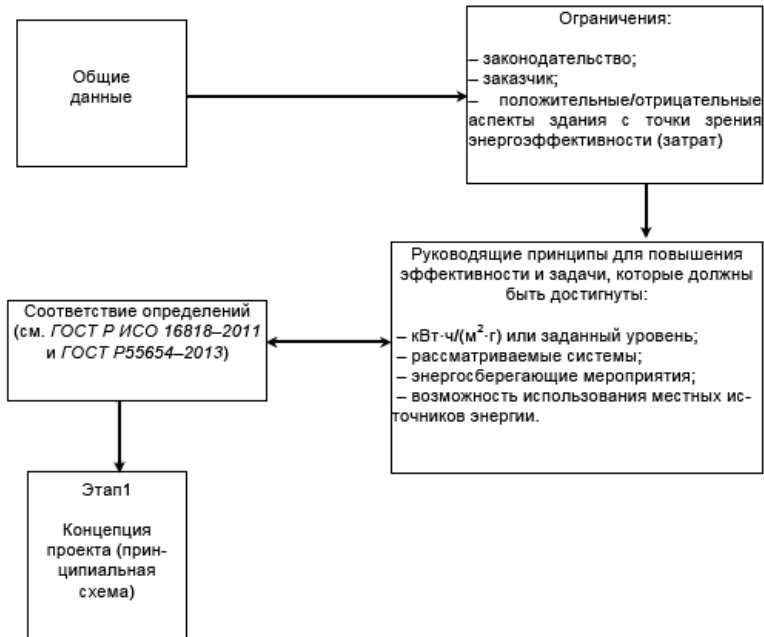
Рисунок А.1 - Блок-схема процесса проектирования энергоэффективности здания
