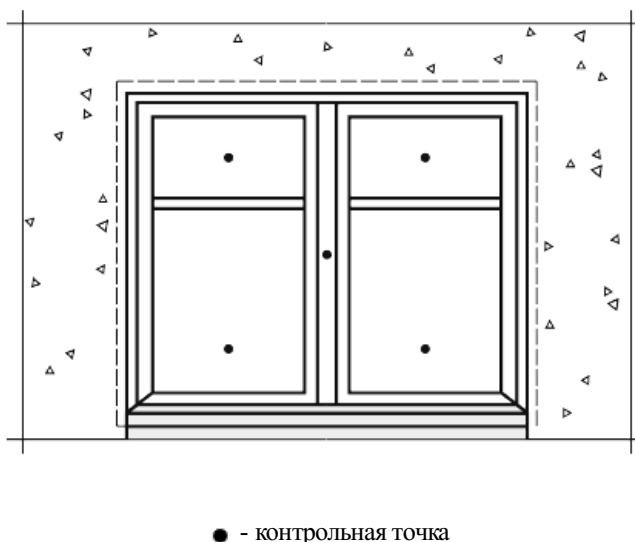
Рисунок Б.7 - Расположение контрольных точек на внешней поверхности окна при измерении вертикальной освещенности (засветки окон)
