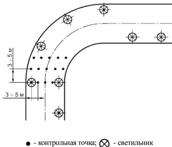
Рисунок Б.6 - Расположение контрольных точек при измерении средней освещенности улиц в местах закругления
