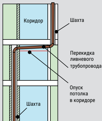
Пример перекидки ливневого трубопровода
