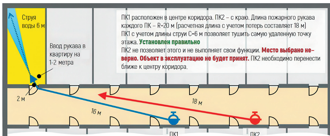
■ Рис. 11. Расчетная длина рукава составляет 18 м, к ней добавляется дальность струи в 6–8 м, что в сумме дает радиус действия пожарного крана
