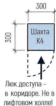
Рис. 19. Пример ошибки размещения лючка доступа к системе K4. Размеры шахты
