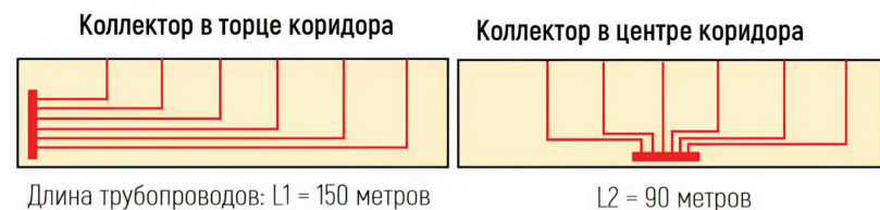
■ Рис. 12. Перенос коллектора из торца коридора в центр приводит к 40 %-ному снижению длин труб
