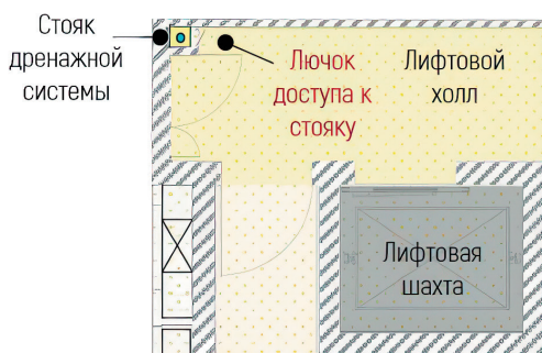
Рис. 19. Пример ошибки размещения лючка доступа к системе K4. Размеры шахты
