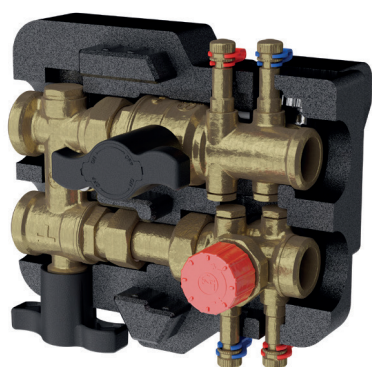
■ Комплект обвязки фанкойлов R280K
