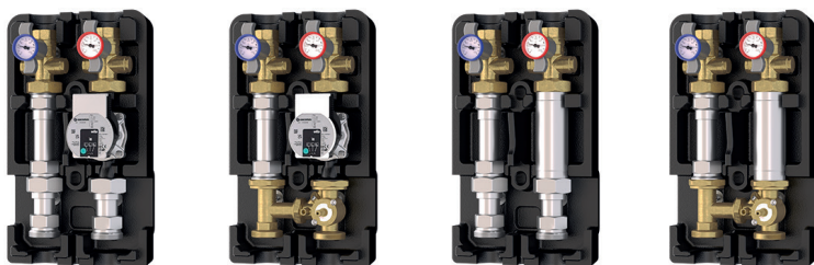
■ Группы быстрого монтажа Giacomini R586R
