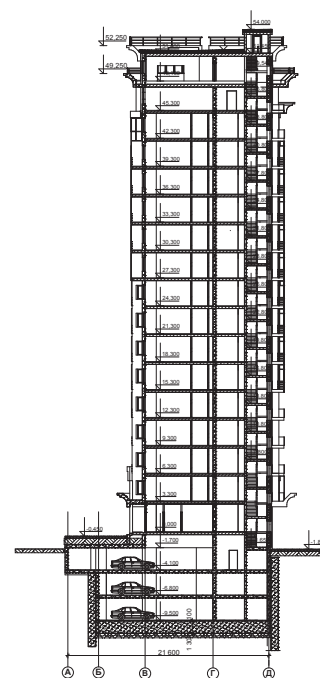
Разрез
