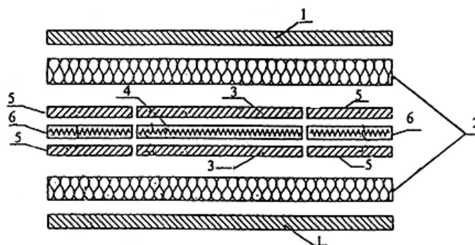
Рисунок А.2 - Схема прибора с двумя тепломерами
