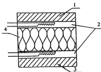
Рисунок А.1 - Схема прибора с одним тепломером
