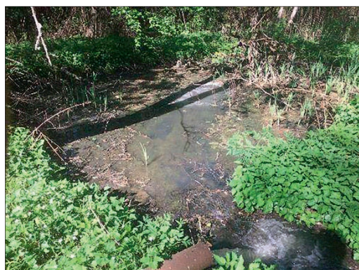
Рис. 1. До установки мобильного очистного сооружения (Милохово, Смоленская область)
