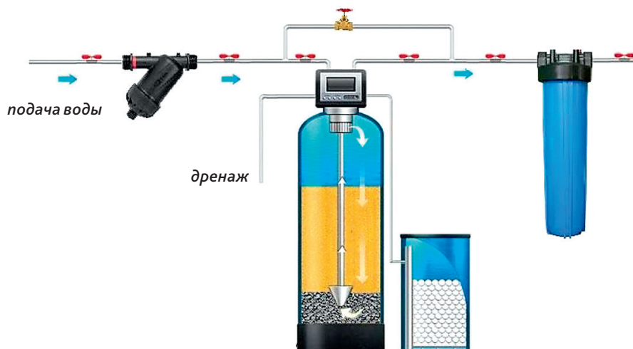
Рис. 3. Схема фильтра-умягчителя циклического действия
