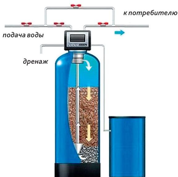
Рис. 2. Сорбционный угольный фильтр
